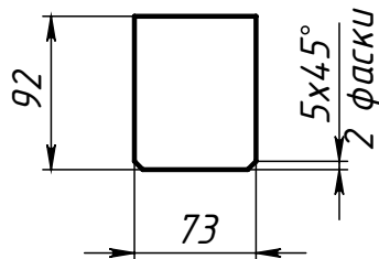
Поз.2 (Ребро)
