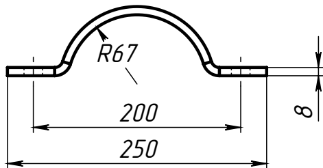
Поз.3 (Хомут)
